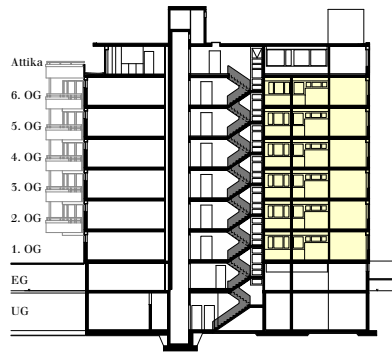
Schnitt
