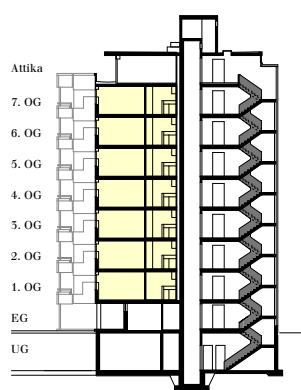
Schnitt
